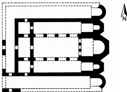
Сл. 16 – Црква у Ђурлинама, основа према Hoddinott-у (преузето: Hoddinott 1963: fig. 104)
