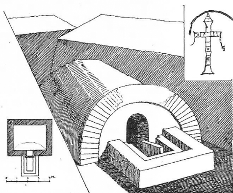
Сл. 25 – Гробница са крстом, према Ф. Каницу (преузето: Каниц 1985: стр. 167)
